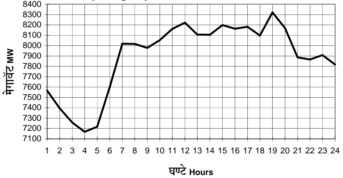
माह नवम्बर 07 में गुजरात का घण्टेवार कॅटर्ड मांग Hourly average Gujarat catered demand for Nov. 2007
