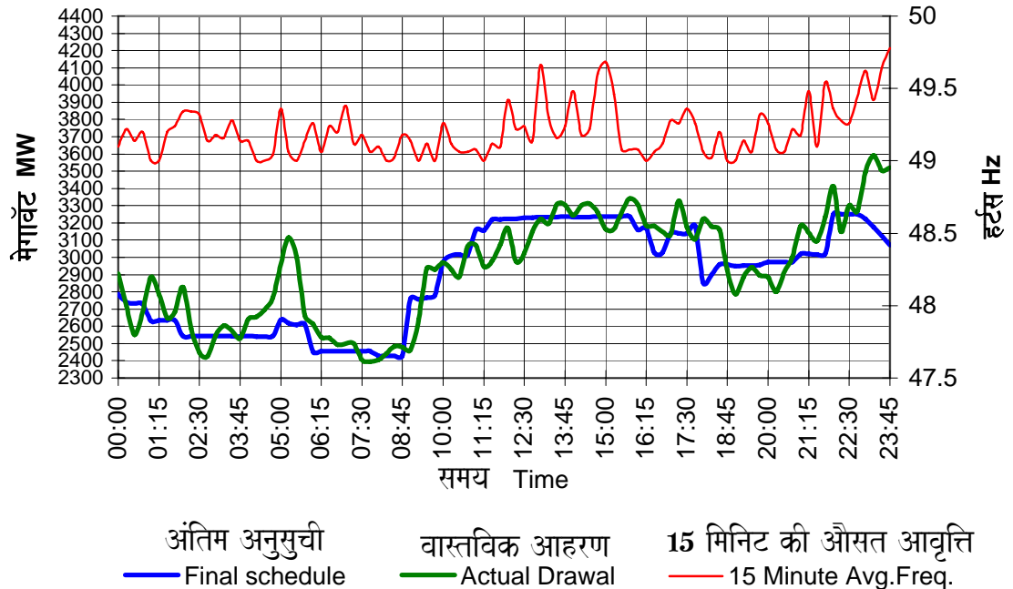
एमएसईबी का 08.11.07 को अनुसूची बनाम वास्तविक आहरण Schedule Vs Actual drawal of MSEB for Date 08.11.07
