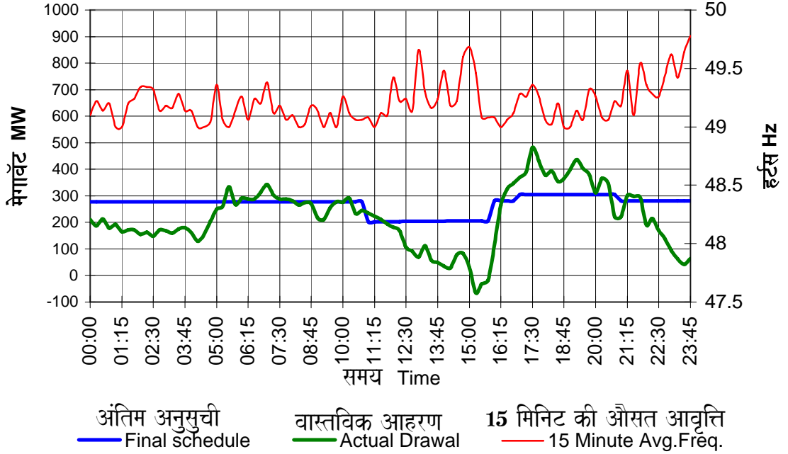
सिएसईबी का 08.11.07 को अनुसूची बनाम वास्तविक आहरण Schedule Vs Actual drawal of CSEB for Date 08.11.07
