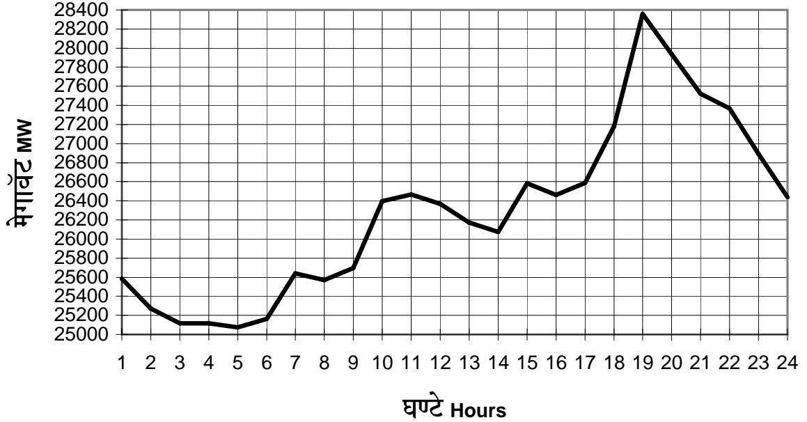
माह नवम्बर 07 में पश्चिम क्षेत्र का घण्टेवार कॅटर्ड मांग Hourly average WR Catered demand for Nov. 2007
