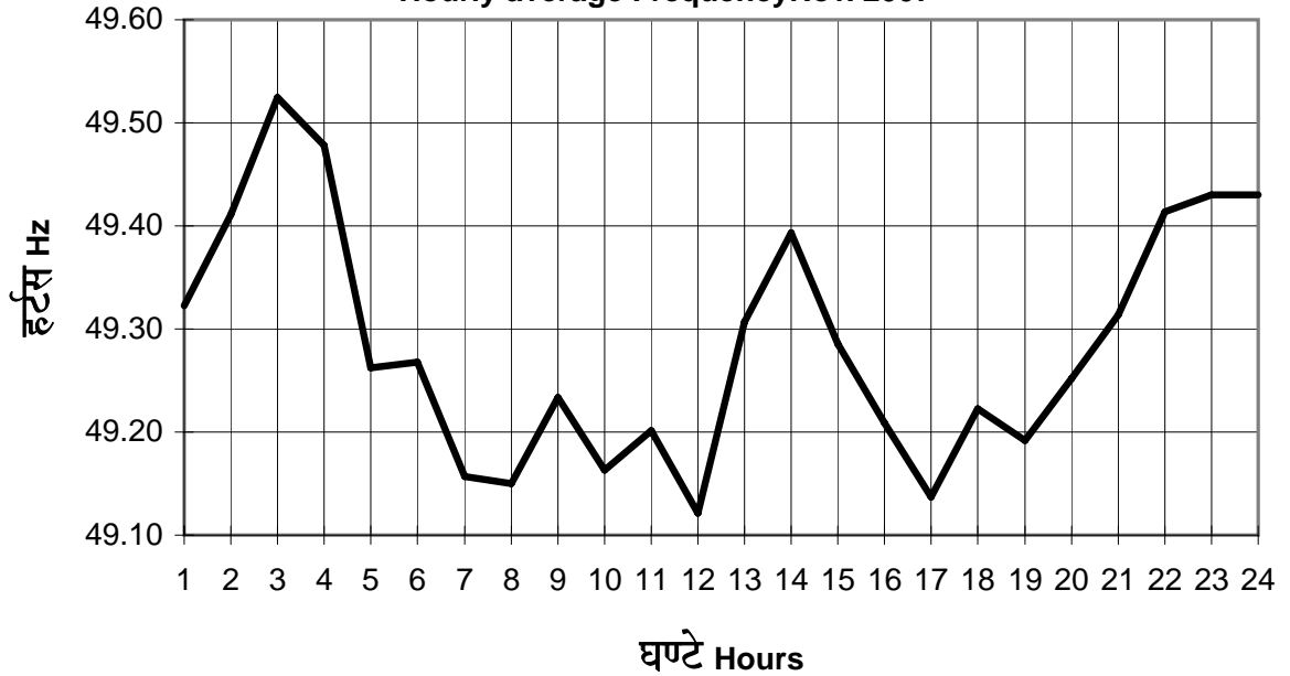
माह नवम्बर 07 में घण्टेवार औसत आवृत्ति Hourly average Frequency Nov. 2007
